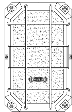
VISTA FRONTAL SIN ACOPLAMIENTO A COLUMNA
