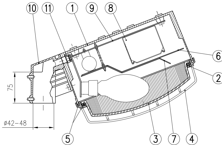
SECCION LONGITUDINAL
