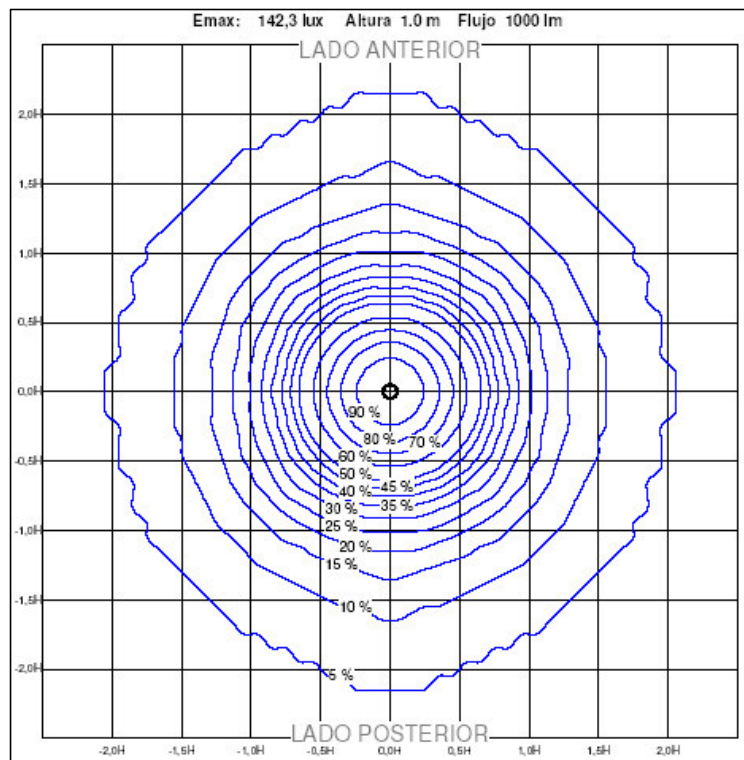
CURVA ISOLUX UNITARIA
