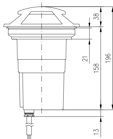
ALZADO
