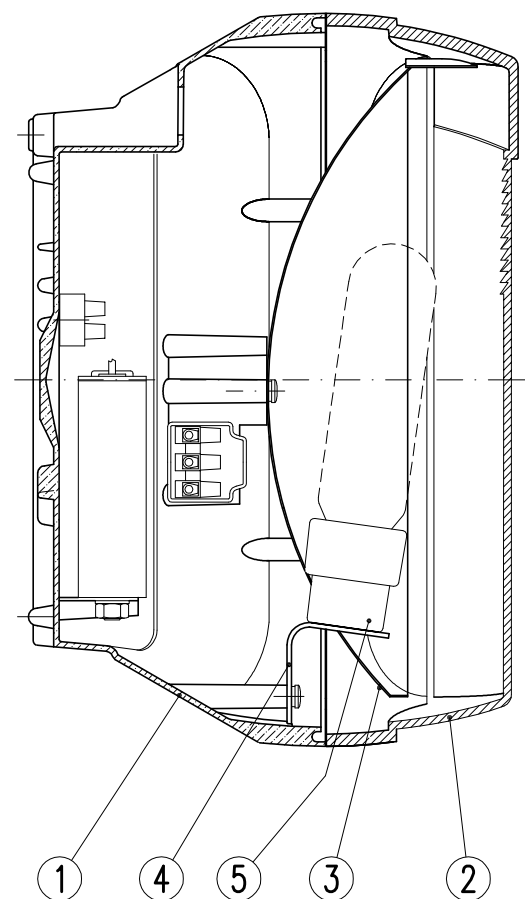
SECCION LONGITUDINAL
