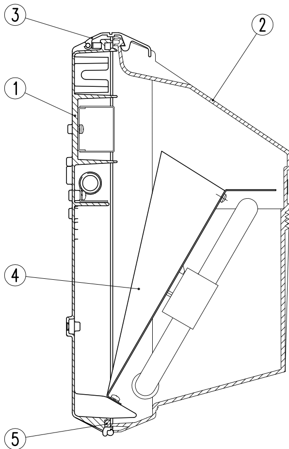
SEMI-SECCIÓN TRANSVERSAL
