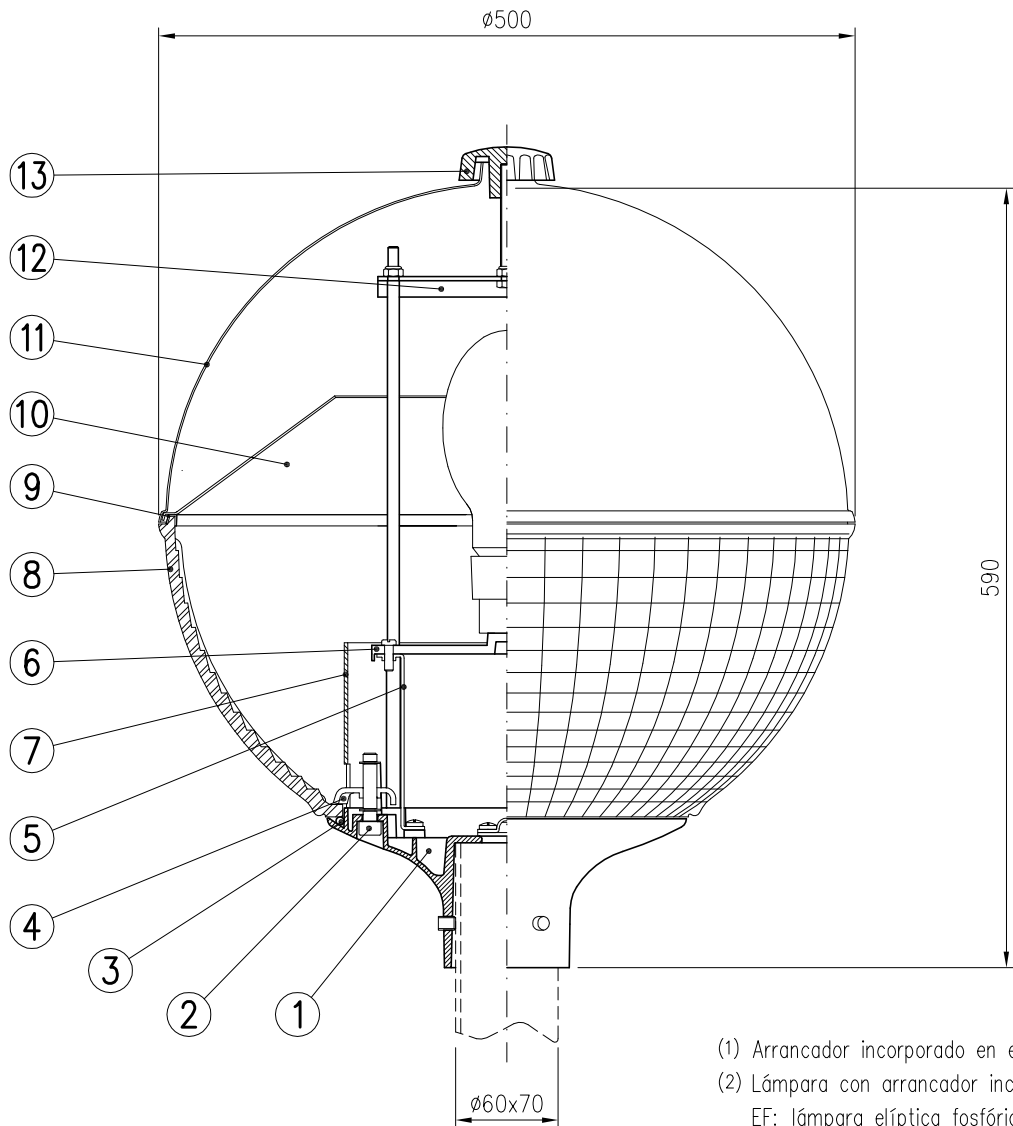
SEMI-SECCION LONGITUDINAL
