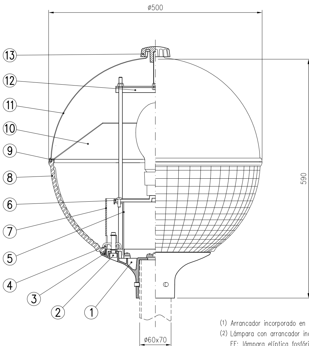
SEMI-SECCION LONGITUDINAL
