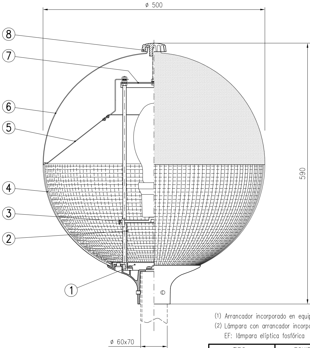
SEMI-SECCION LONGITUDINAL
