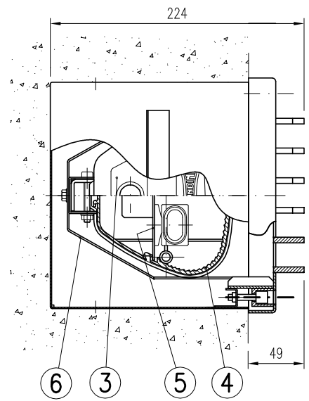
SEMI-SECCION TRANSVERSAL
