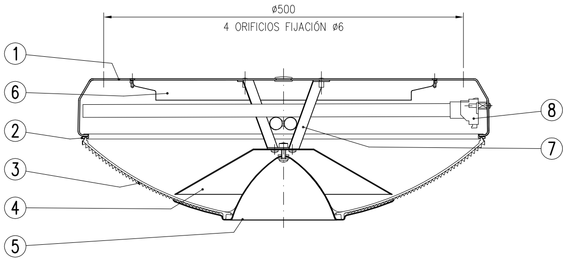
SECCIÓN TRANSVERSAL
