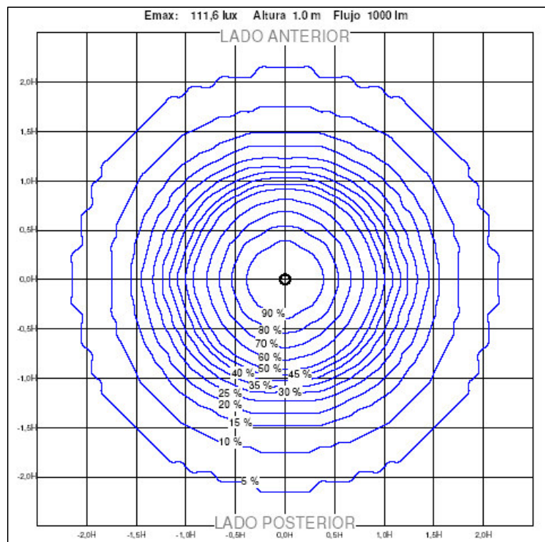
CURVA ISOLUX UNITARIA
