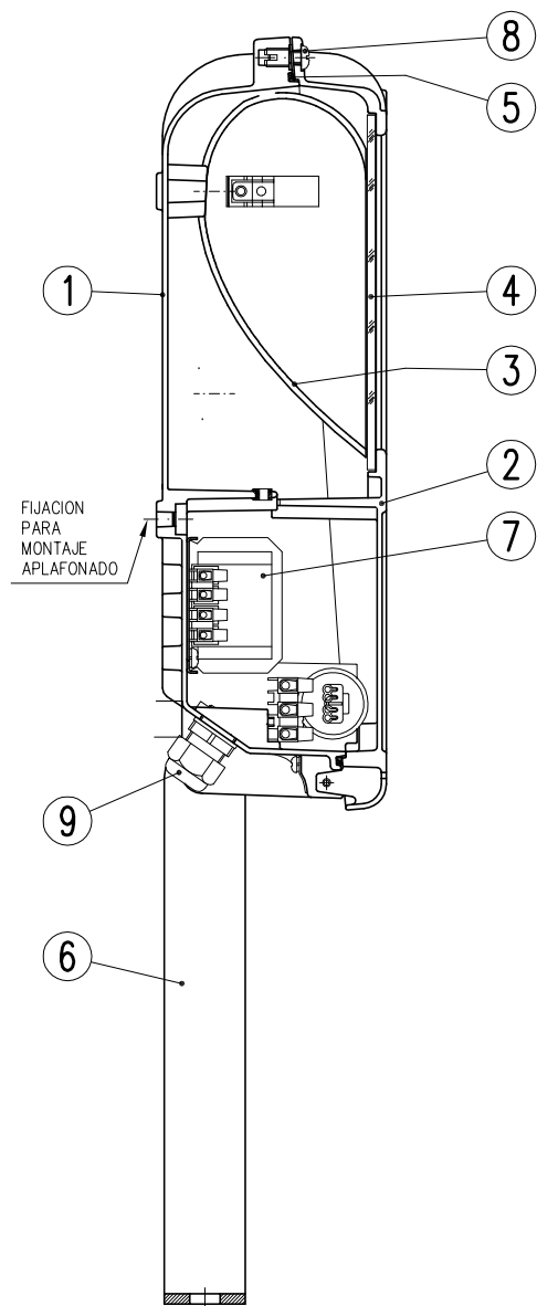
SEMI-SECCIÓN TRANSVERSAL
