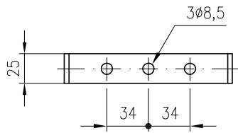
HORQUILLA FIJACION
