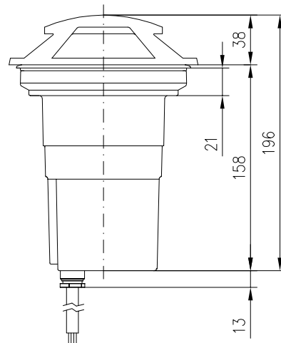
ALZADO
