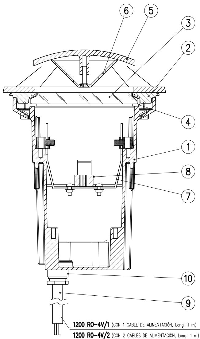
SECCION LONGITUDINAL
