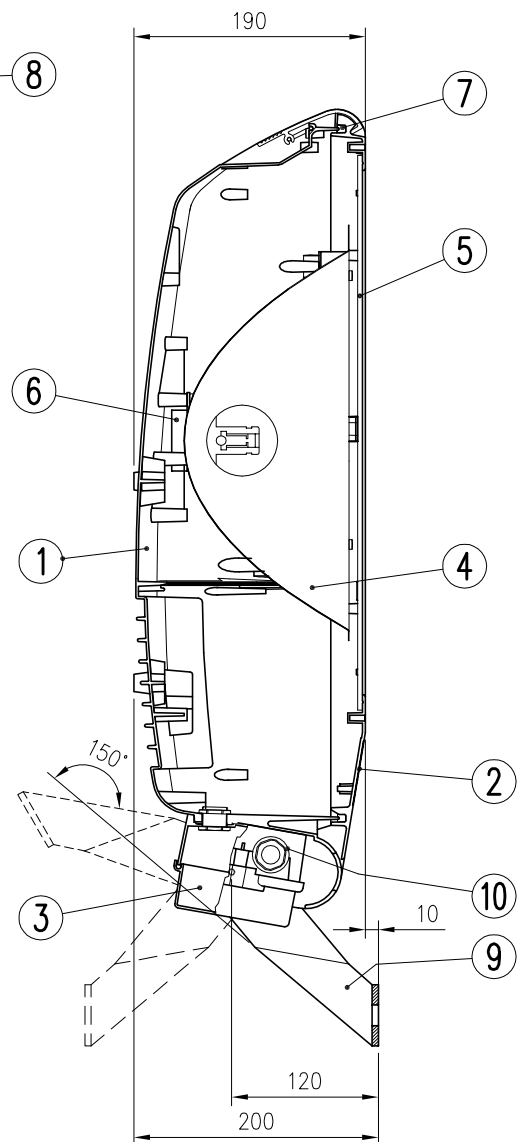
SECCION LONGITUDINAL
