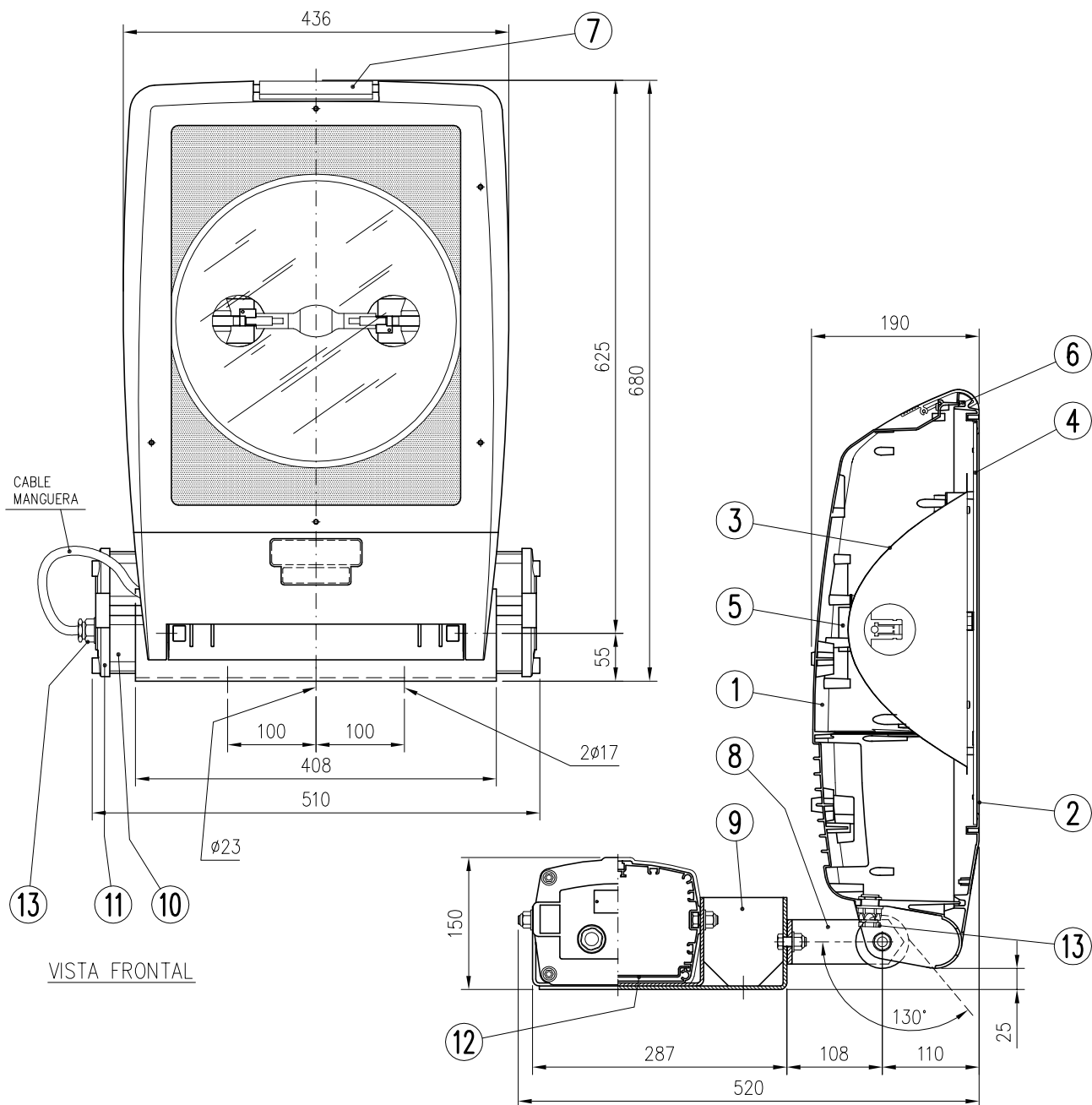
SECCION LONGITUDINAL
