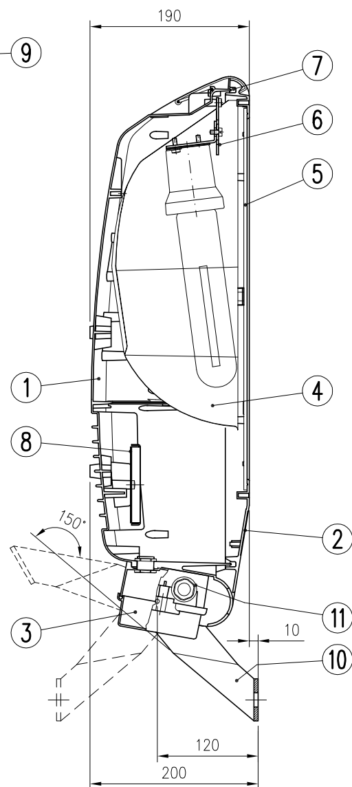
SECCION LONGITUDINAL
