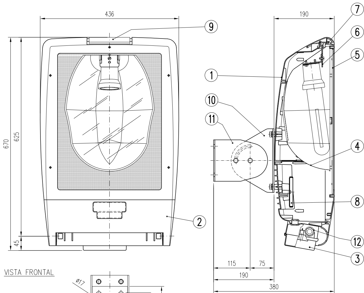
SECCION LONGITUDINAL
