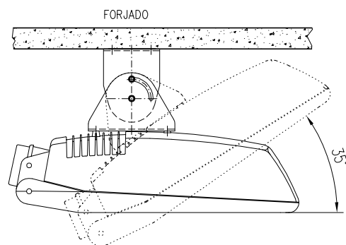
ORIENTACIONES ADMISIBLES, SEGÚN EL SISTEMA DE MONTAJE
