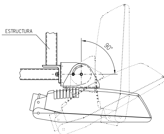
ORIENTACIONES ADMISIBLES, SEGÚN EL SISTEMA DE MONTAJE
