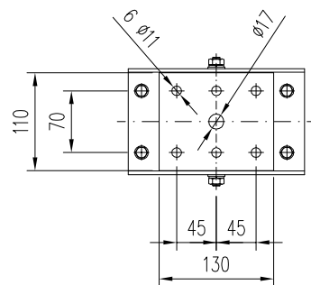
HORQUILLA FIJACIÓN CONJUNTO
