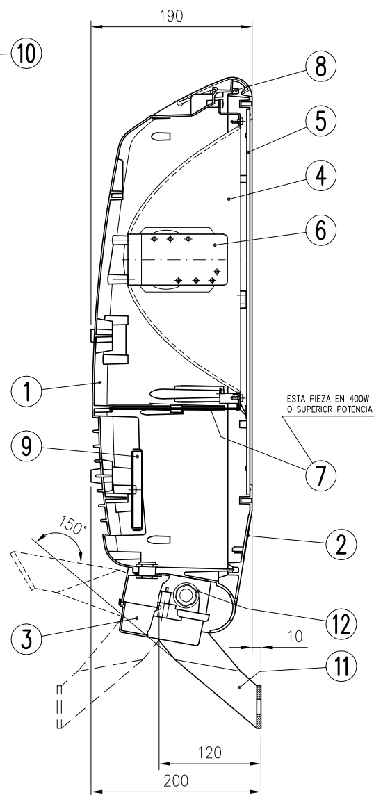
SECCION LONGITUDINAL
