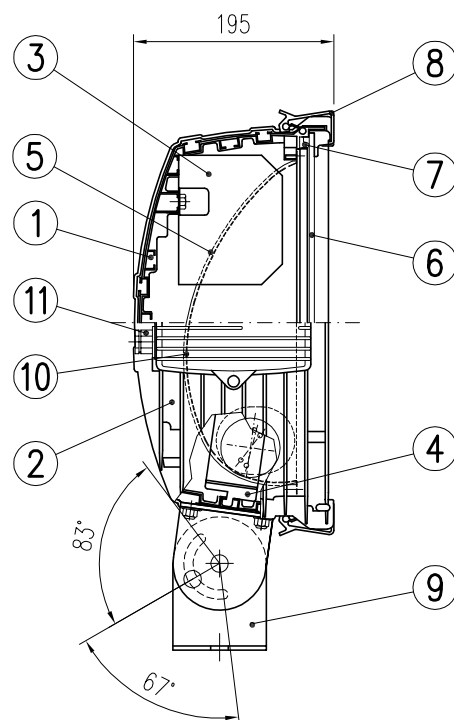
SEMI SECCION LATERAL
