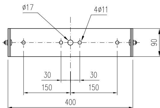
HORQUILLA FIJACIÓN
