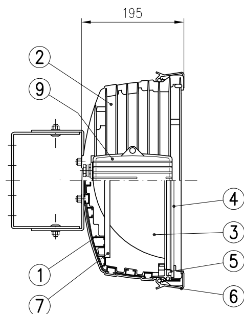
SEMI SECCION LATERAL
