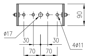
HORQUILLA DE FIJACION
