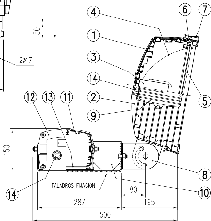
SECCION LONGITUDINAL
