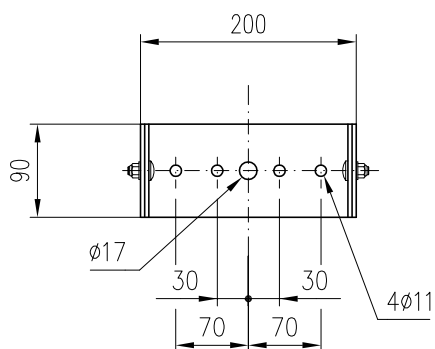
HORQUILLA FIJACIÓN
